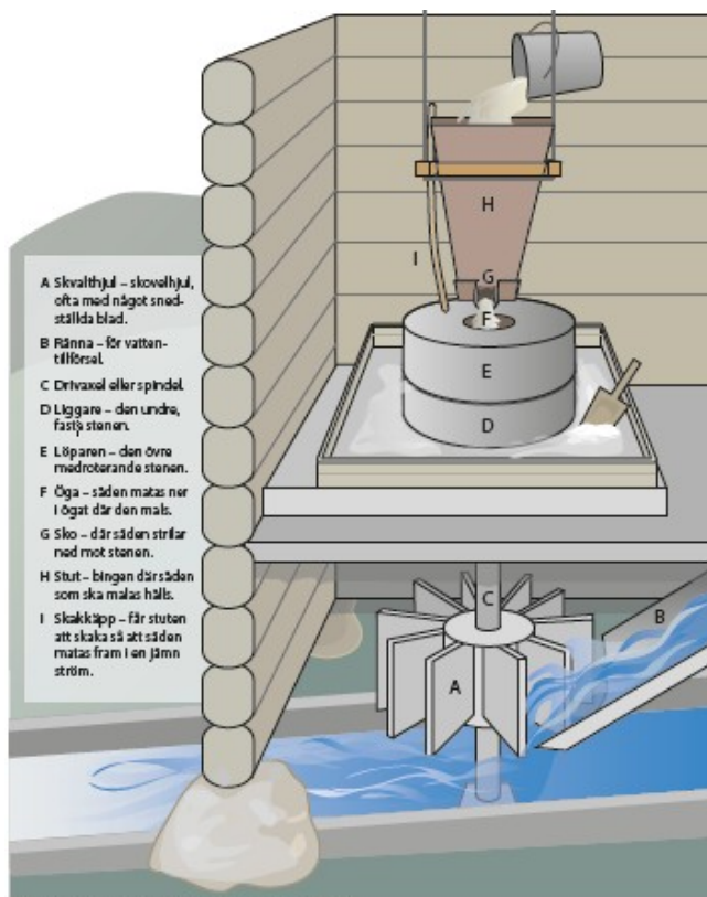
Principskiss av skvaltkvarn. Illustration: Gunilla Guldbbrand, 2018
