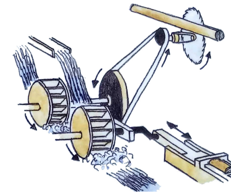
Kraftöverföringen till cirkelsåg och spånhyvel vid Torvsjö kvarnar Bild: Erik Axelsson, Skogs- och samemuseet Lycksele
