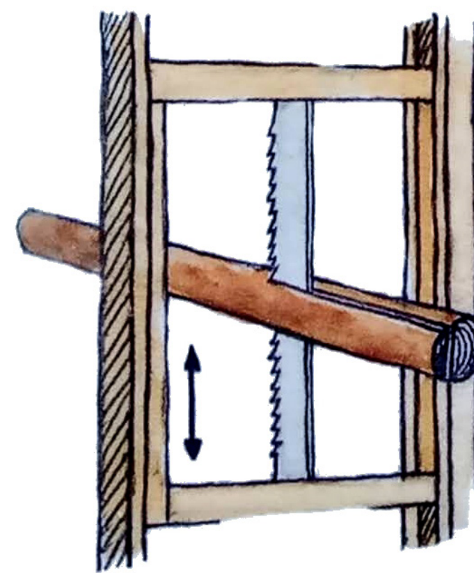
Princip för ramsågens arbetssätt. Bild: Från skylt vid Torvsjö kvarnar Erik Axelsson, Skogs- och samemuseet Lycksele
